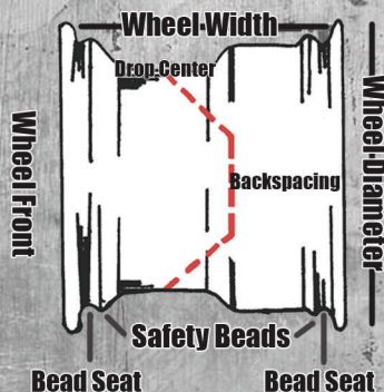
4 - Lug Bolt Pattern Center to Center
